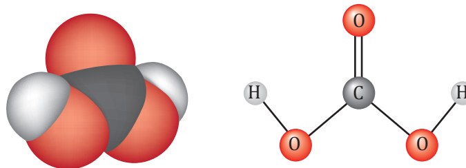
Modelo molecular del ácido carbónico (H 2 CO 3 )
